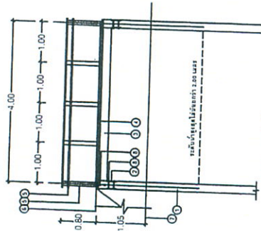
แบบรูปตัดตามขวาง
