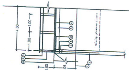
แบบรูปตัดมอดับริม
